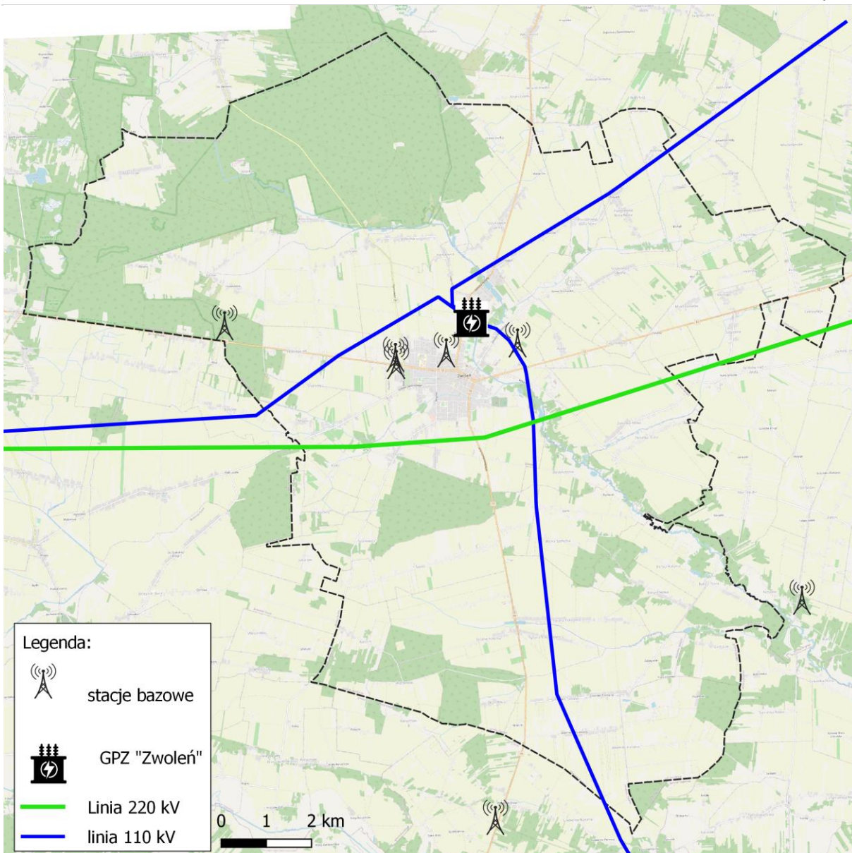
Rysunek 3. Lokalizacja stacji bazowych telefonii komórkowej oraz linii energetycznych wysokiego napięcia na tle gminy Zwoleń
